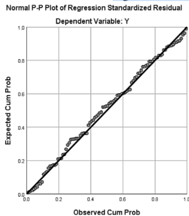
Gambar 1. Uji Normalitas
